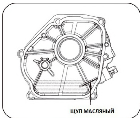
Рисунок 2. Проверка уровня моторного масла.
