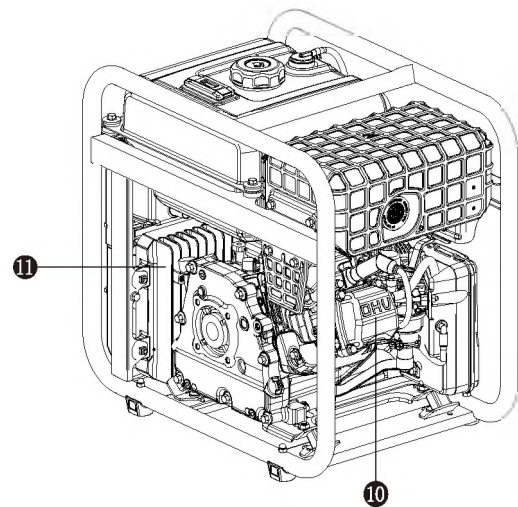
Рисунок 1а. Расположение основных узлов и элементов управления.
