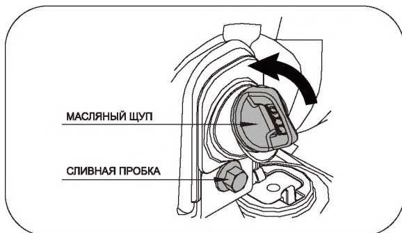
Рисунок 6. Расположение масляного щупа и сливной пробки.
