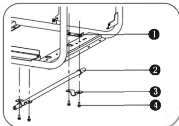
Рисунок 1. Монтаж колесной оси генераторной установки.
